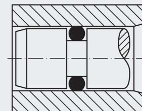
Radiaal geperst, aan de buitenzijde afdichtend
