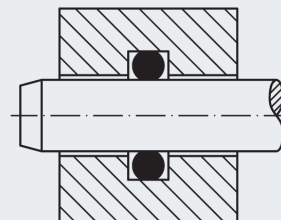
Radiaal geperst, aan de binnenzijde afdichtend
